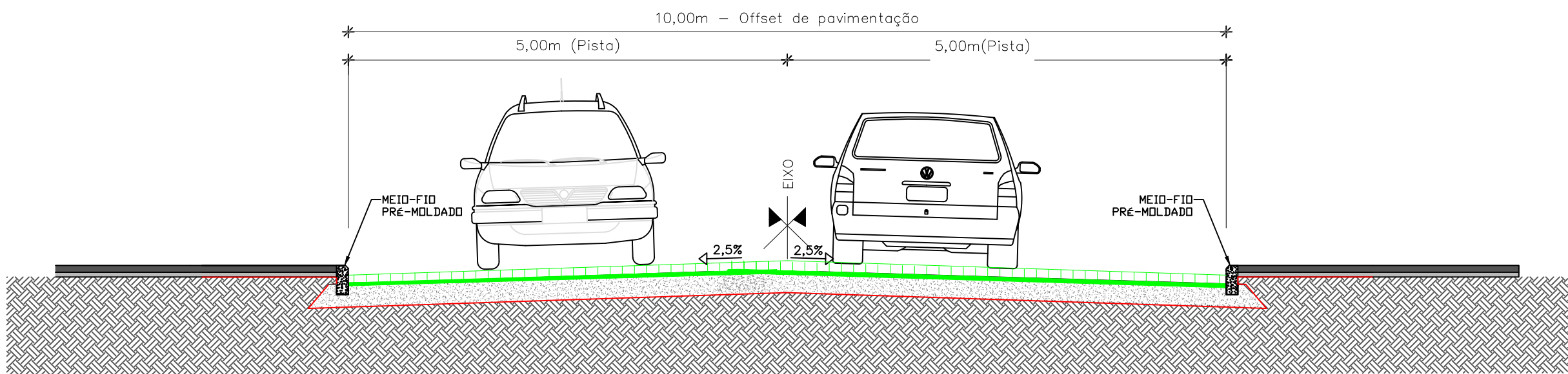
SEÇÃO TIPO DE PAVIMENTAÇÃO- Offset de pavimentação com bloco intertravado-RUA CONS. TEODORO ALBRESCHT
